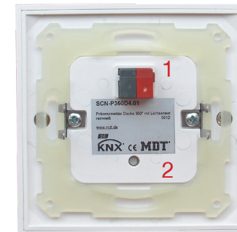
SCN-P360x4.03 Rückansicht - Back view
